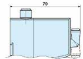
Schwenkwinkel mit Steckanschluss Rohrleitung 4 mm AD
