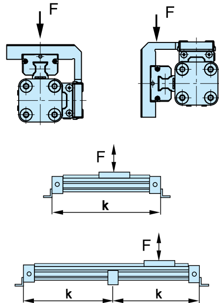
Belastungsfall 1 Schlitten oben
