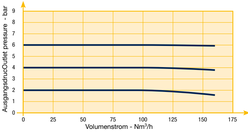
Fließkurve 1"
