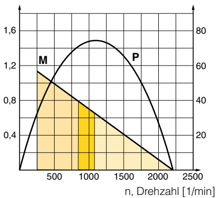
P1V-P007**2200
