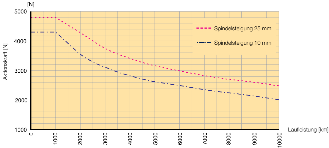
HMRS18 Laufleistung / Aktionskraft
