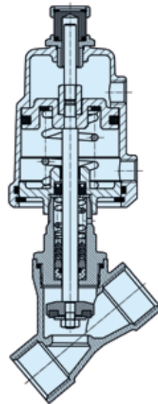
Stromlos geöffnetes Ventil
