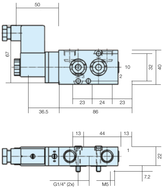
Abmessungsangabe Nr. 3
