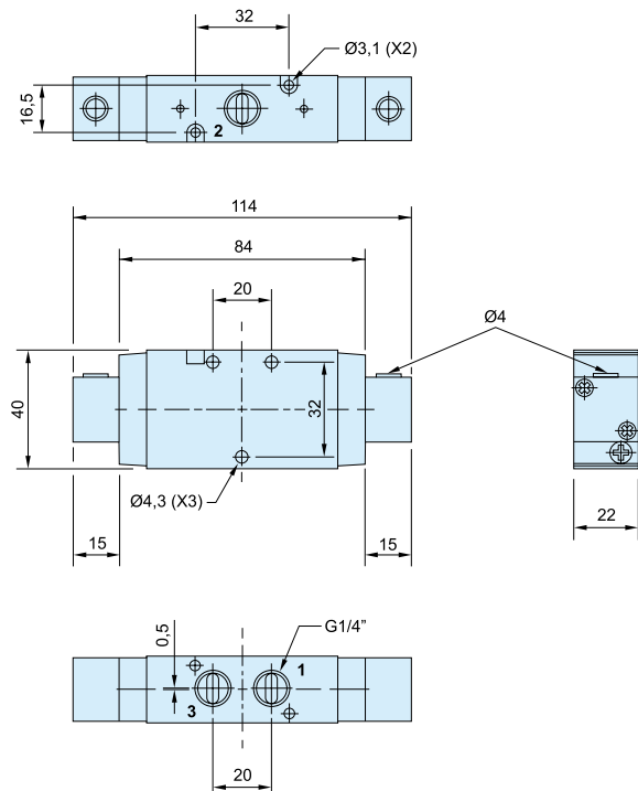
P2LBZ 3/2 Pneumatisch/Pneumatisch
