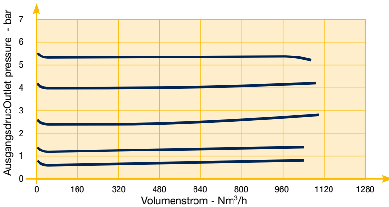
Fließkurve 2"
