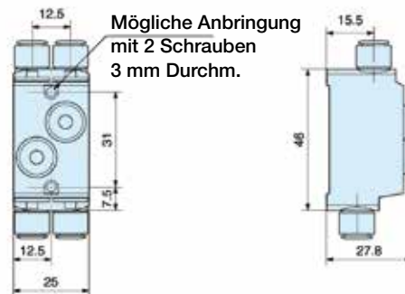
Mögliche Anbringung mit 2 Schrauben 3 mm Durchm.
