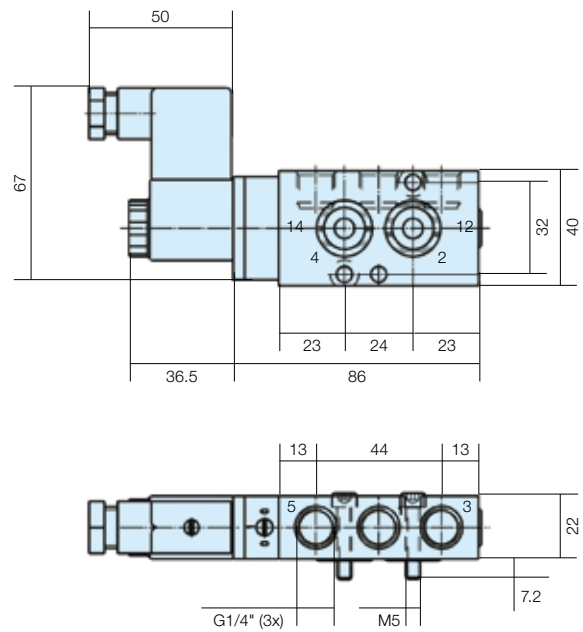
Abmessungsangabe Nr. 4
