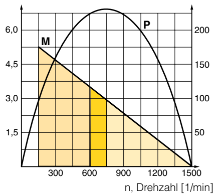
P1V-P023**1500
