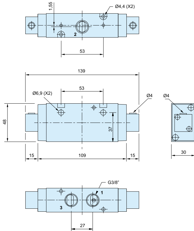
P2LCZ 3/2 Magnetventil/Magnetventil
