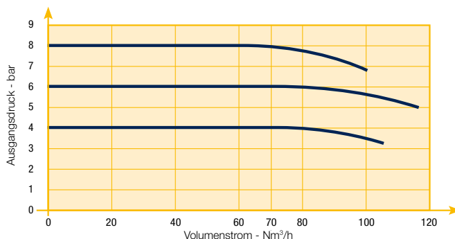
Volumenstromkurve 1/4"
