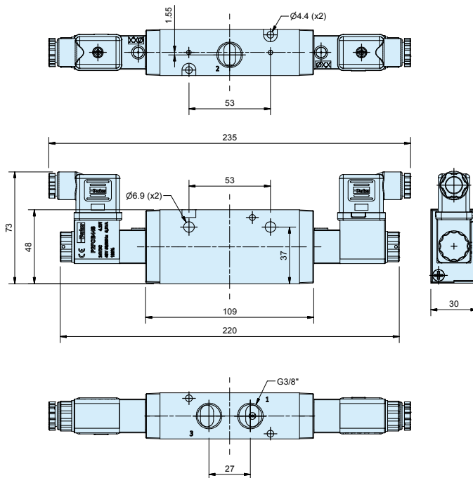
P2LCZ 3/2 Magnetventil/Magnetventil
