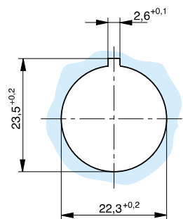
Einbauausschnitt \varnothing 22 mm
