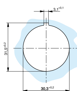
Einbauausschnitt \varnothing 30 mm
