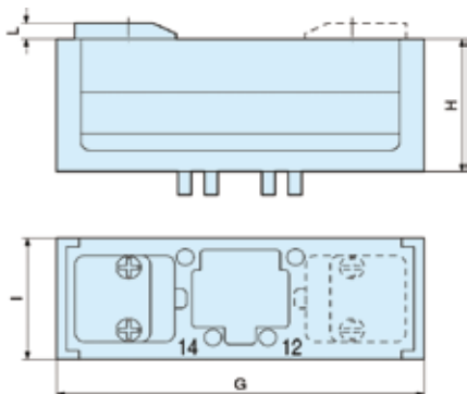
Pneumatisch betätigt
