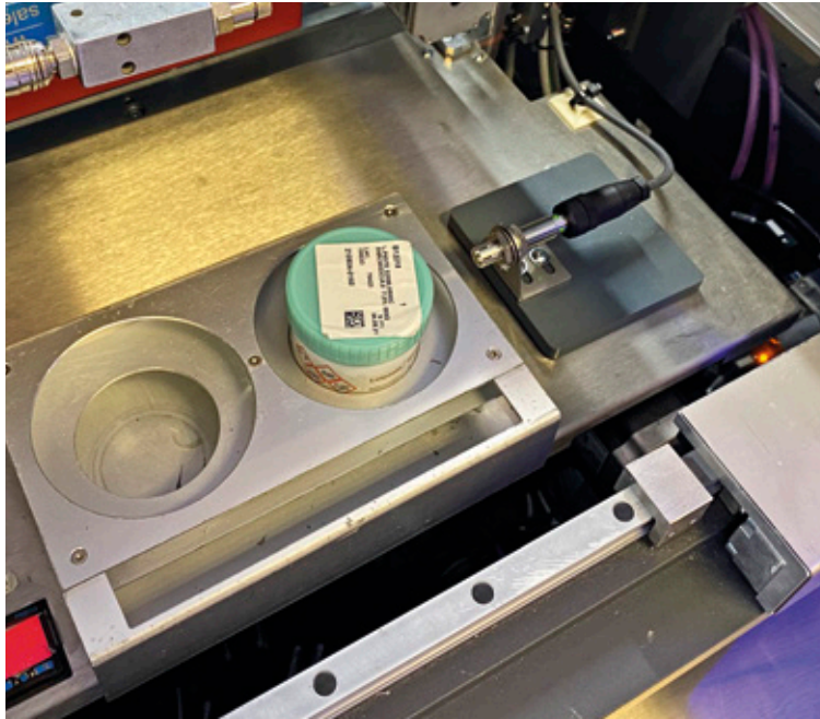
Turcks Condition-Monitoring-Sensor CMTH erfasst in den Lotpastendruckern Temperatur und Luftfeuchte und überträgt die Werte an seinen IO-Link-Master
