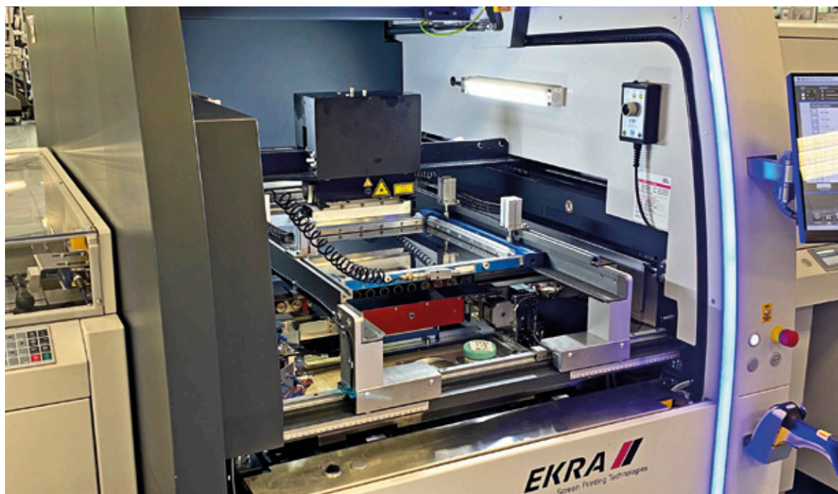
Im vorderen Bereich des Druckers werden die Lotpasten eingesetzt, der CMTH-Sensor erfasst direkt daneben die Umgebungsbedingungen
