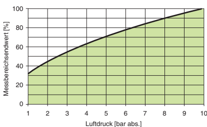
Funktionsbereich LDS 1000 GAPL
