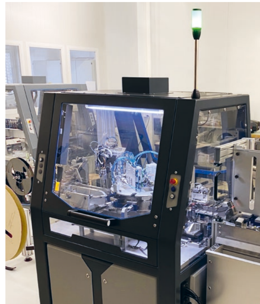
Un module machine d'Aatec, éclairé à l'intérieur par des lampes de machines Banner. Visible à tous, la tour de signalisation de Banner placée tout en haut indique l'état de la machine.
